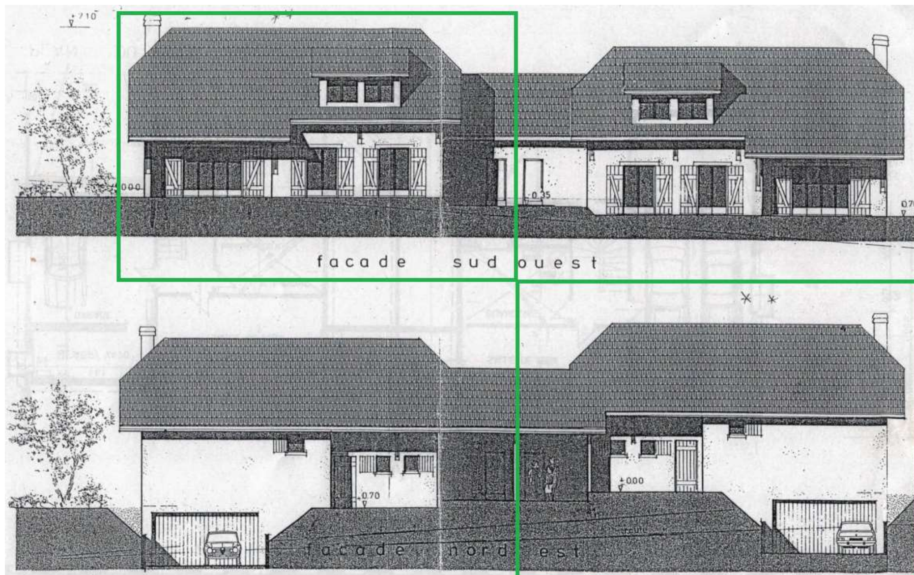
Plans de la maison avant l'extension de 2002
